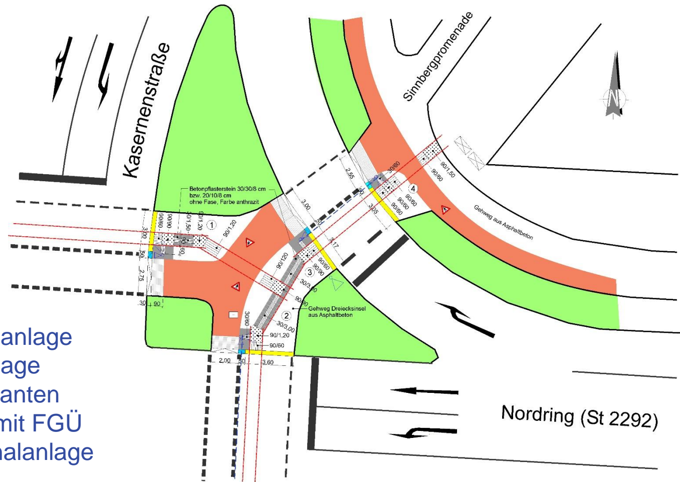
Barrierefreie Querungsstellen mit Bodenindikatoren (Lageplan-Auszug Bad Kissingen 2009)
